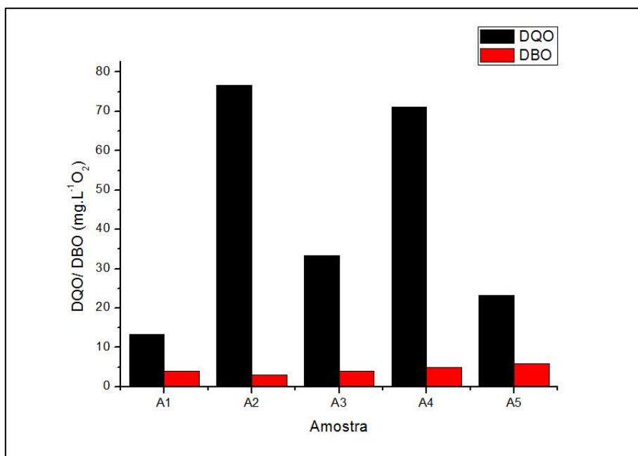
Gráfico 3. Dados experimentais DQO e DBO das cinco amostras
