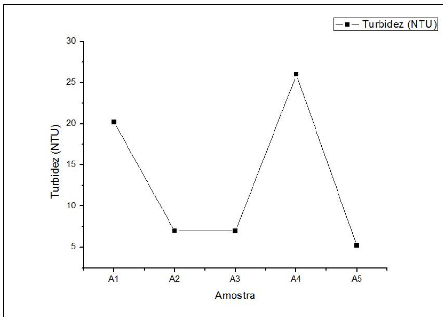
Gráfico 2. Resultados das análises de turbidez para as cinco amostras
