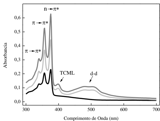
Figura 3. Espectros de UV-vis das soluções 1 \times 10^{-6} \text{ mol L}^{-1} do ligante TSAB e dos complexos metálicos Cu(II)-TSAB e Cu(II) 2 -TSAB em THF (ligante TSAB linha preta, Cu(II)-TSAB linha cinza claro e Cu(II) 2 -TSAB linha cinza escuro).
